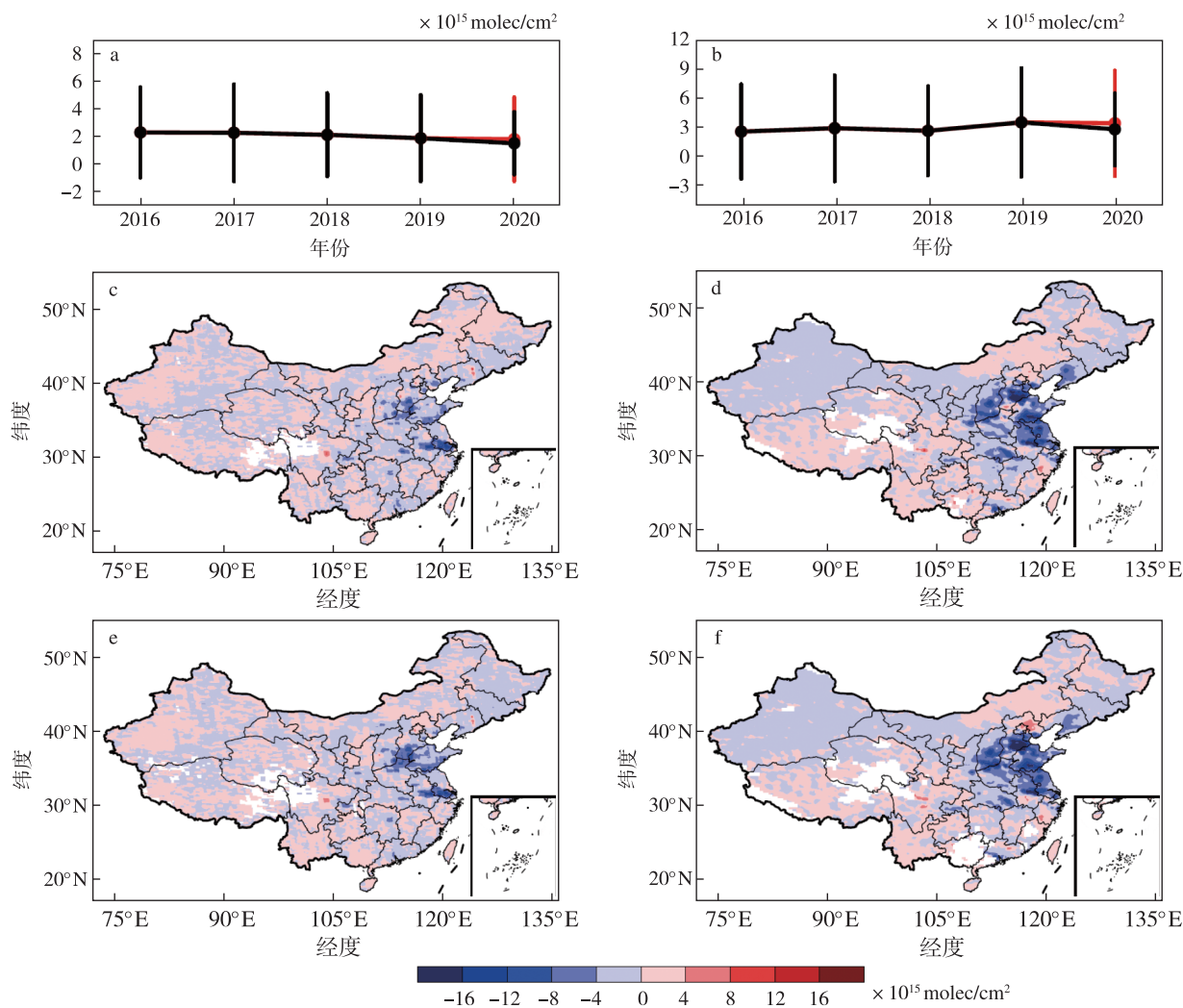
图3 疫情期间 OMI(a,c,e)和 GOME-2(b,d,f)反演的 NO 2 柱浓度的变化:(a,b)2016—2020 逐年平均 2—3 月的 NO 2 变化(黑线是实际观测;2020 年红点根据 2016—2019 年 2—3 月 NO 2 的线性外推结果;误差条代表不同格点 NO 2 的范围);(c,d)2020 年 NO 2 相对于预期的变化;(e,f)2020 年 NO 2 相对于 2019 年同期的变化
