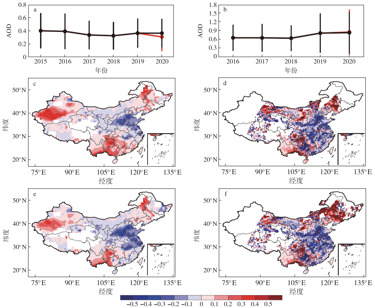
图5 疫情期间 MODIS(a,c,e)和葵花8号(b,d,f)反演的气溶胶光学厚度(AOD)的变化:(a,b)2016—2020 逐年平均 2—3 月的 AOD 变化(黑线是实际观测;2020 年红点根据 2016—2019 年 2—3 月 AOD 的线性外推结果;误差条代表不同格点 NO 2 的范围);(c,d)2020 年 AOD 相对于预期的变化;(e,f)2020 年 AOD 相对于 2019 年同期的变化
